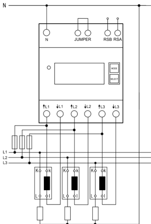
Koblingskjema TN
