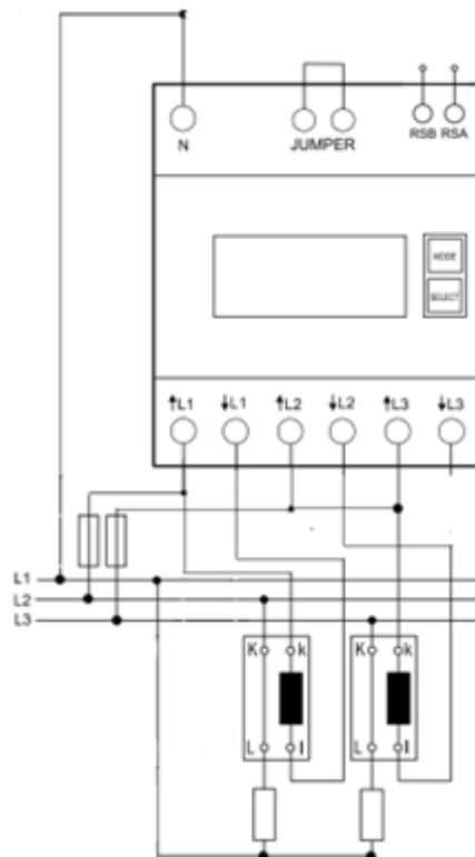
Koblingskjema IT
